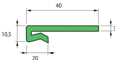
Perfil P 40 - verde P 40 Profile - green Profil P 40 - vert
